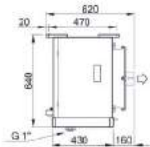
SERIE FR Ø 400
