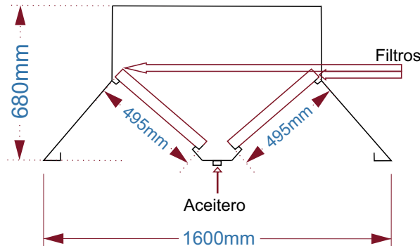
CAMPANA CENTRAL CON PLENUM
